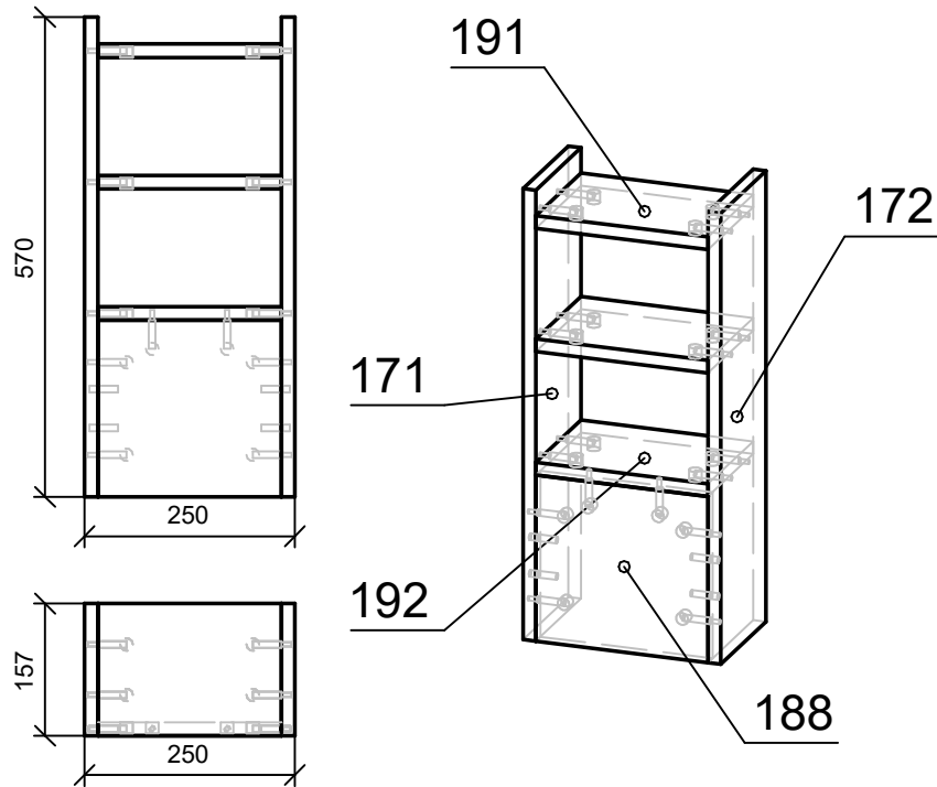
Спецификация на панели
