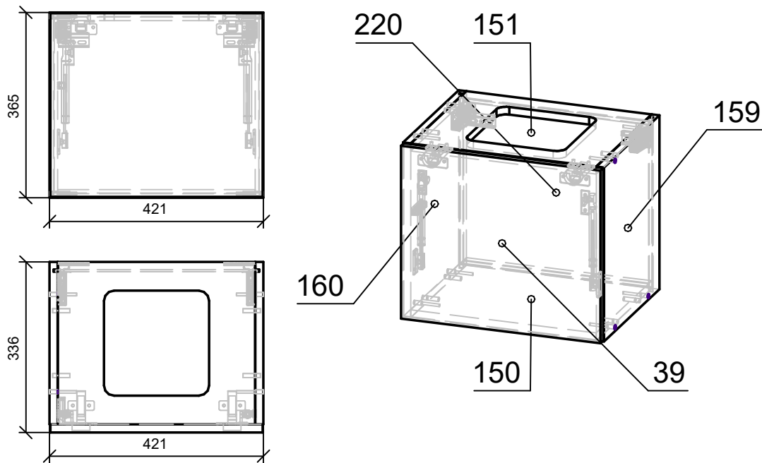
Спецификация на панели
