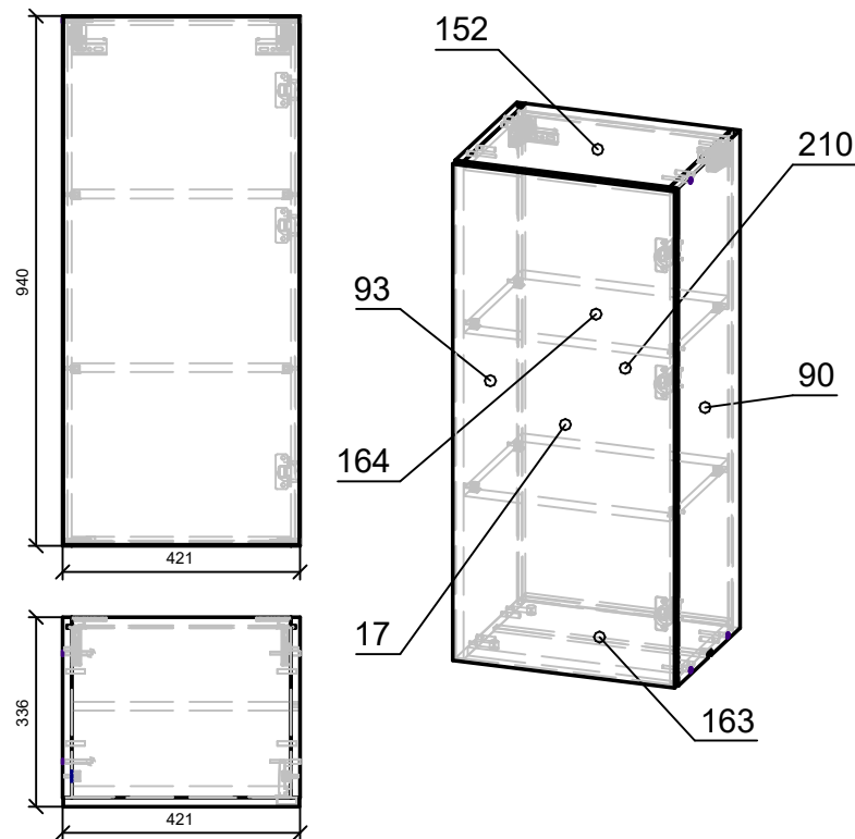
Спецификация на панели
