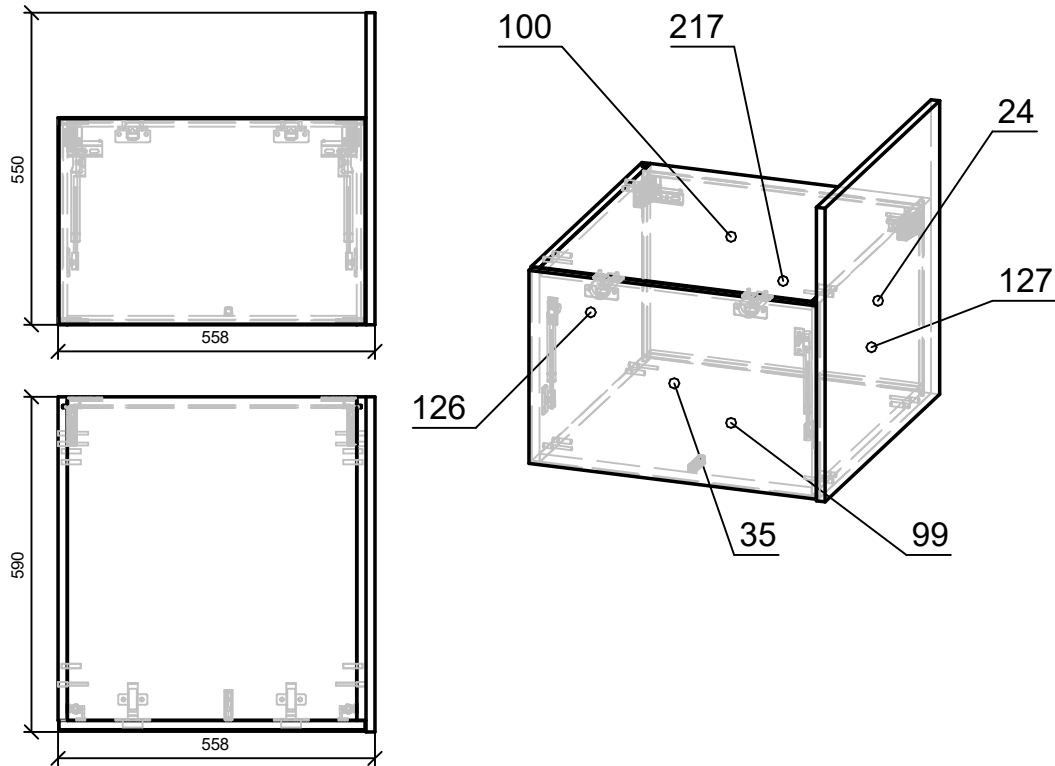
Спецификация на панели
