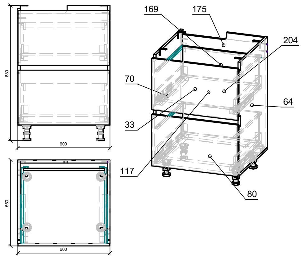
Спецификация на панели
