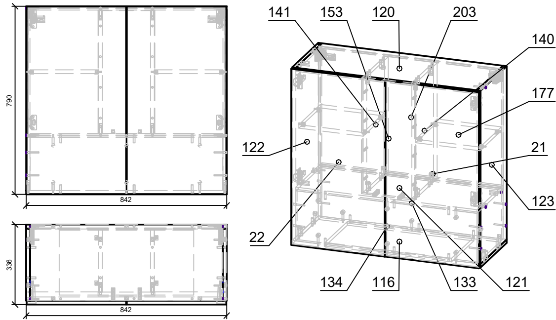
Спецификация на панели
