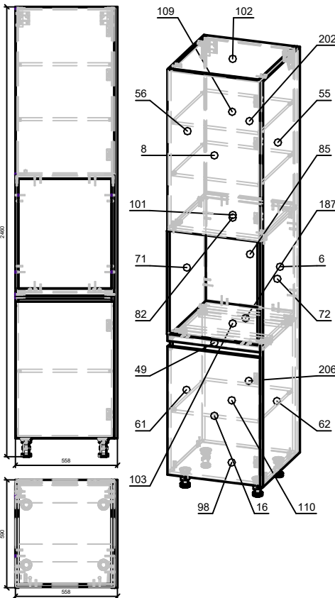
Спецификация на панели
