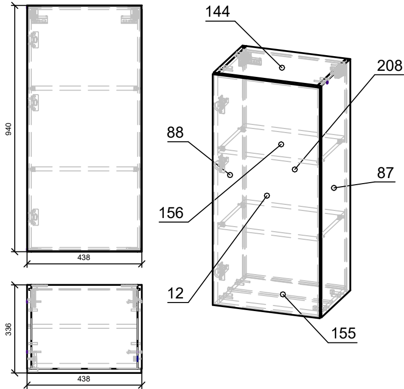
Спецификация на панели
