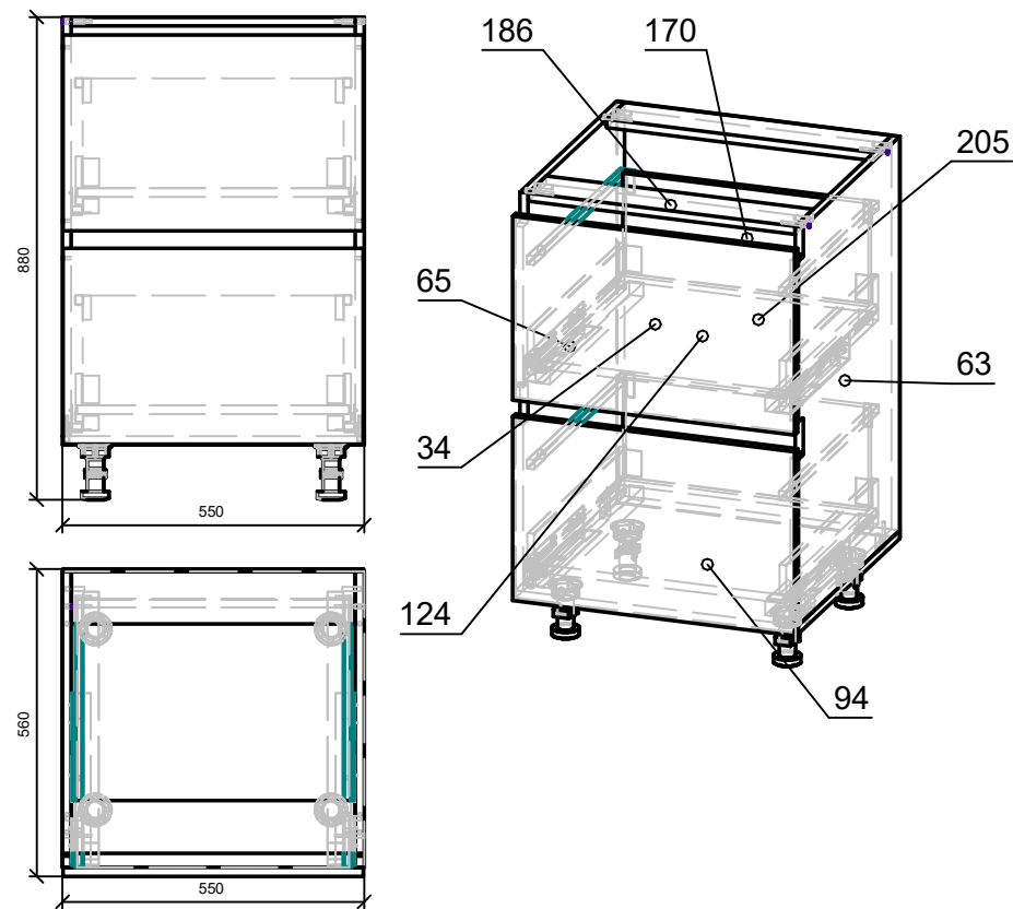
Спецификация на панели
