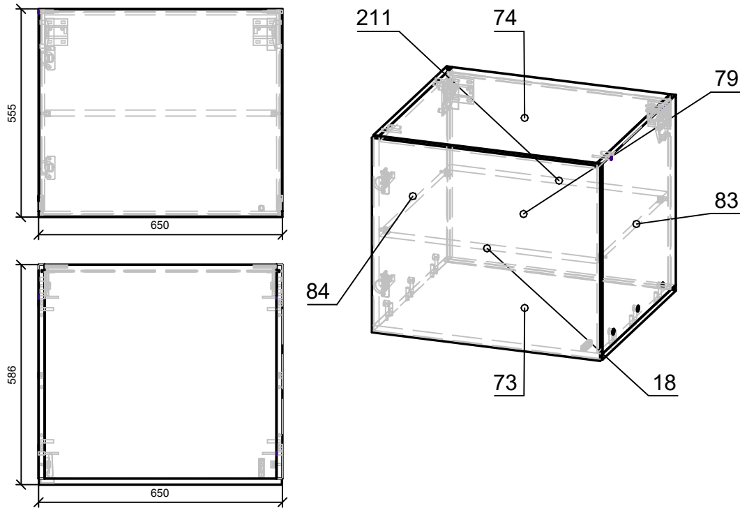
Спецификация на панели
