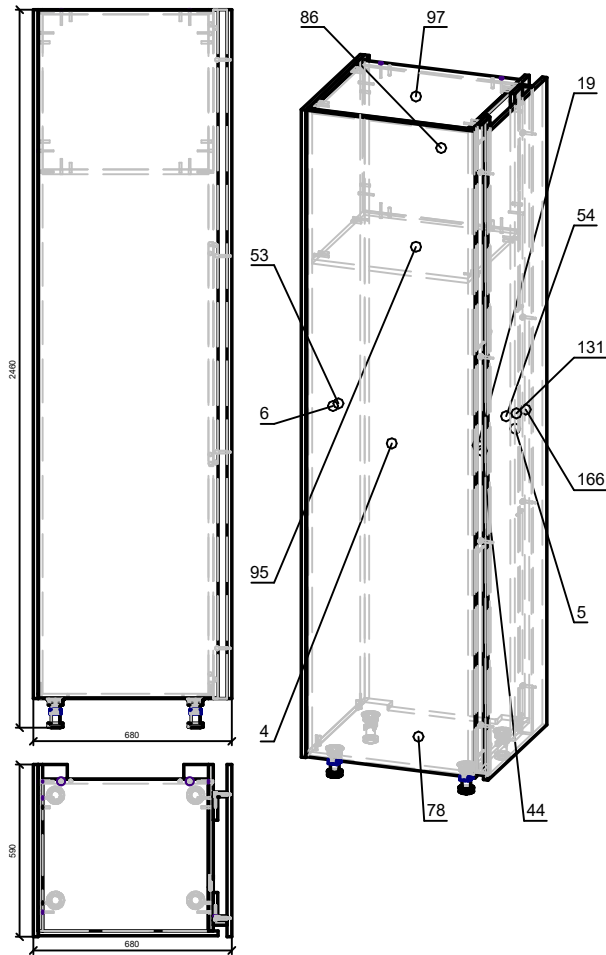
Спецификация на панели
